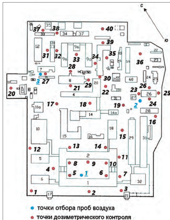
Схема дозиметрического контроля на промплощадке Московского филиала
