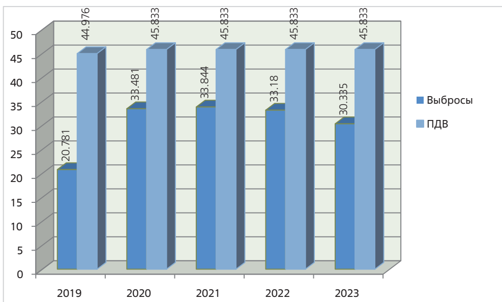
Диаграмма 4. Динамика изменения выбросов вредных химических веществ (тонн/год)
